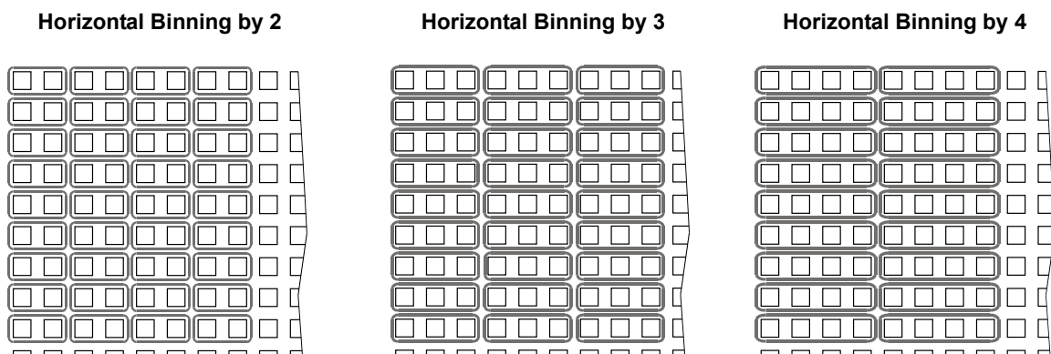
Fig. 66: Horizontal Binning
