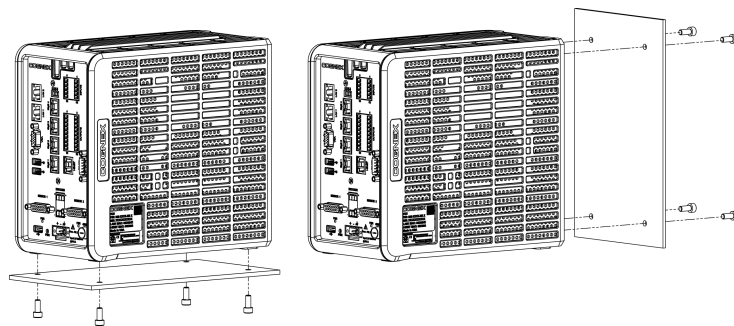
图 2-1: 安装视觉控制器
