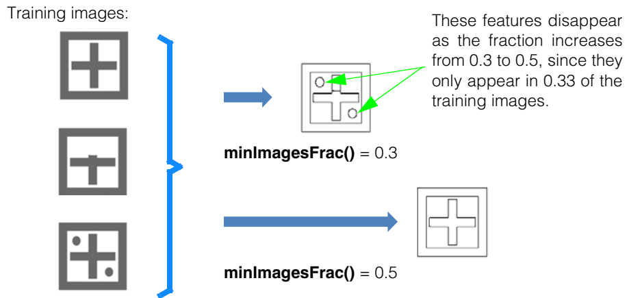
Figure 342. Using the minImagesFrac() parameter
